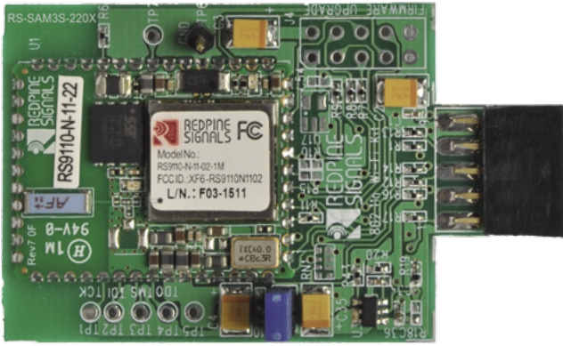
Fotografia 8. Zestaw RS-SAM3S-220X Wi-Fi add-on card for SAM3S-EK
